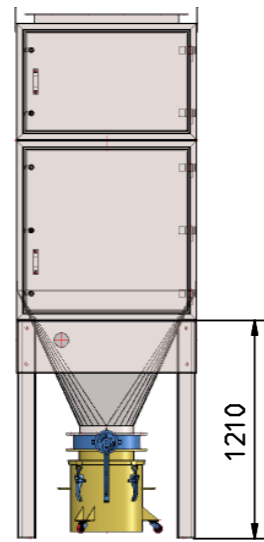
② Staubsammeltopf 45 Ltr. mit Absperrklappe DN 300 Dust bin 45 ltr. with butterfly valve DN 300
