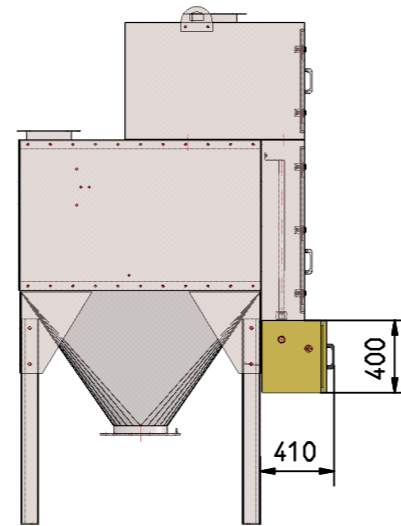
⑥ Schutzgehäuse für Abreinigungssystem Protective housing for cleaning system
