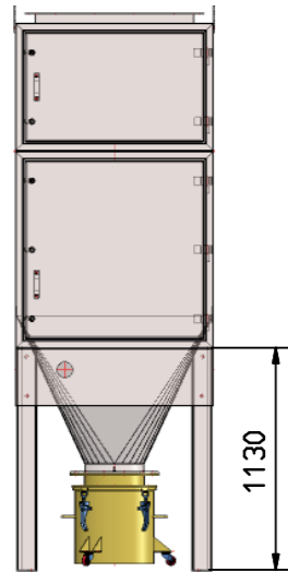
① Staubsammeltopf 45 Ltr. Dust bin 45 ltr.
