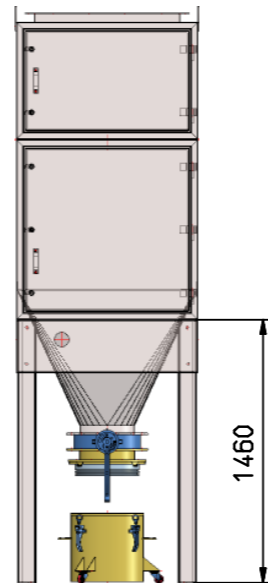
③ Staubsammeltopf 45 Ltr. mit Safe-Change und Absperrklappe DN 300 Dust bin 45 ltr. with Safe-Change and butterfly valve DN 300
