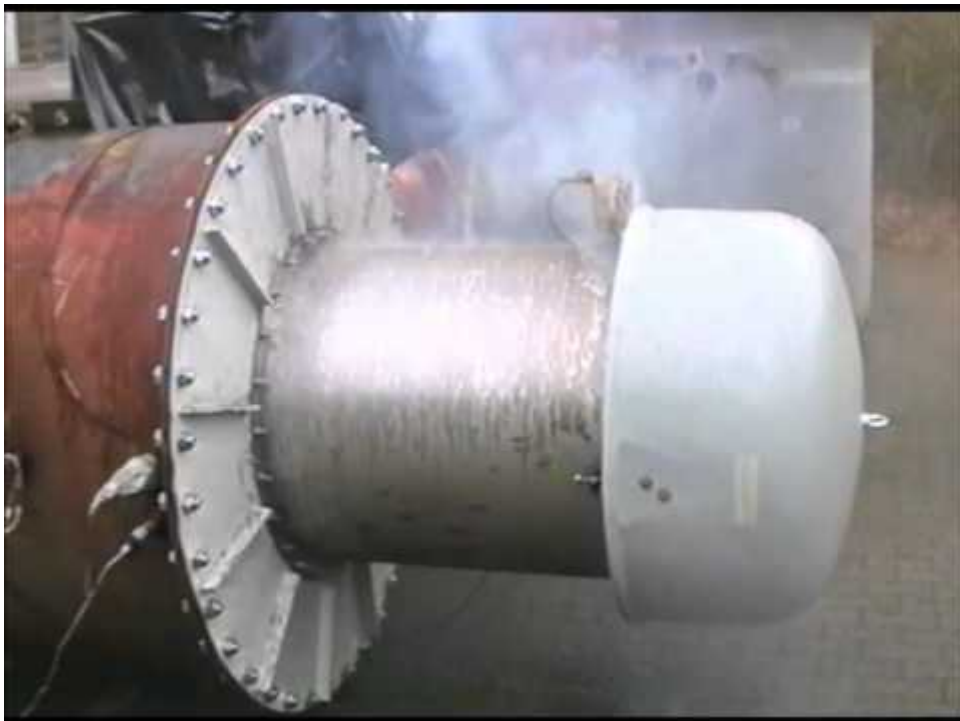
Siloaufsatzfilter INFA-JETRON Typ AJB wird in Explosionsversuchen auf Druckstoßfestigkeit getestet.
